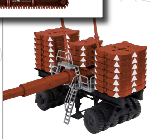
Ballastwagen / ballast trailer
